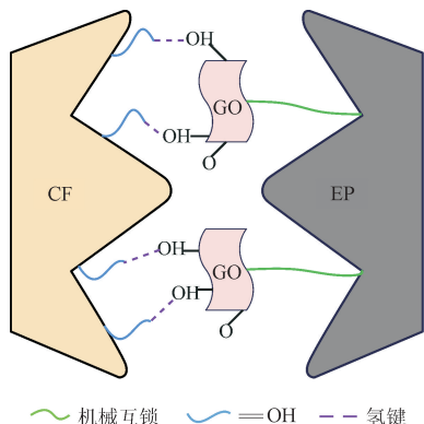
图 14 GO-CF 增强复合材料的界面增强机理示意图
