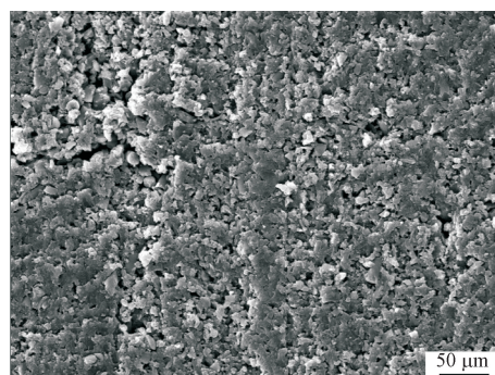
图9 GO质量分数为0.5%时的SEM图
