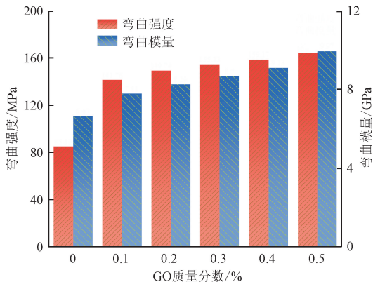
图 13 不同 GO 质量分数的 GO-CF 编织复合材料试验弯曲强度及弯曲模量
