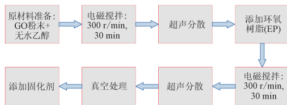
图1 含 GO 的混合溶液制备核心过程流程
