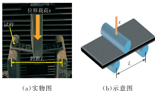
图3 三点弯曲测试实物及示意图
