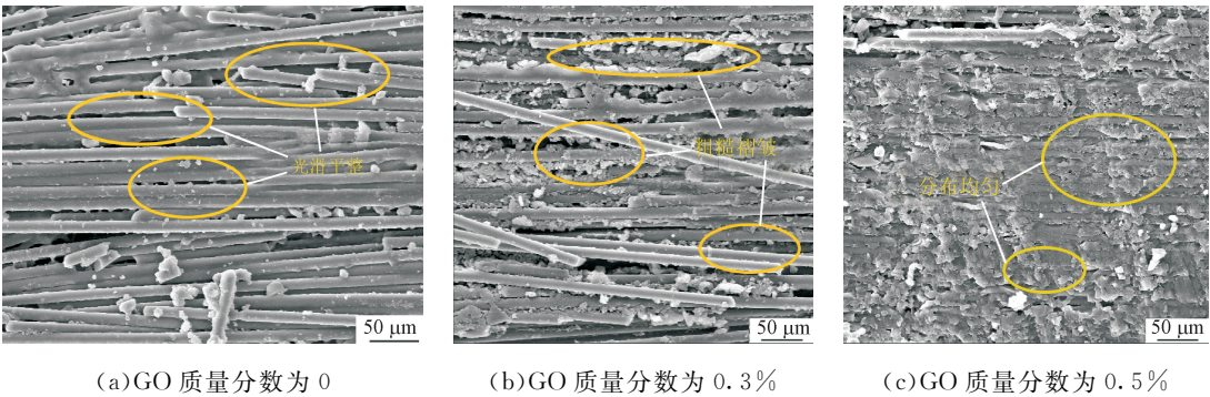
图 10 不同 GO 质量分数的复合材料微观表面形貌图
