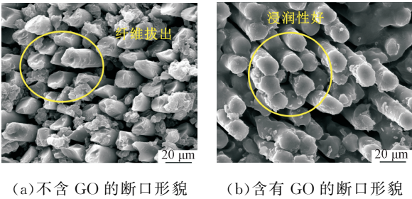
图 11 不同 GO 质量分数的复合材料断口形貌图
