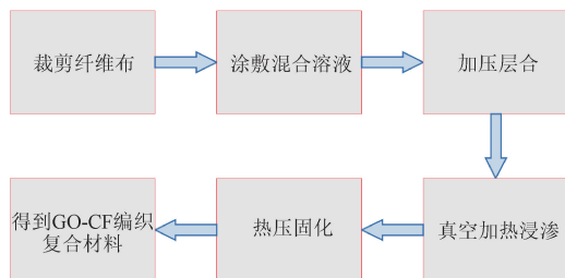
图2 GO-CF 增强编织复合材料制备流程图
