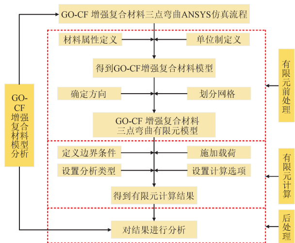
图 4 基于 ANSYS 三点弯曲仿真流程
